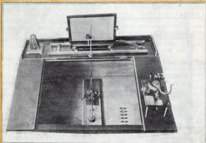
Телеграф Якоби
