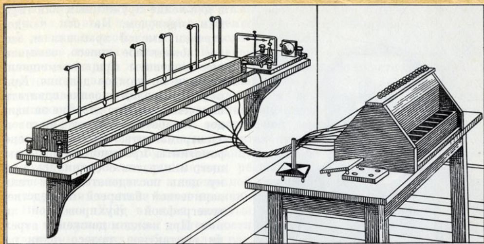
Телеграф Шиллинга
