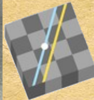
Евклидова геометрия
